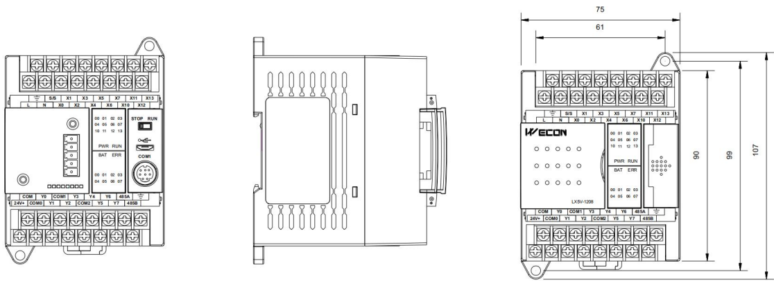
LX5S 1208 安装尺寸图
