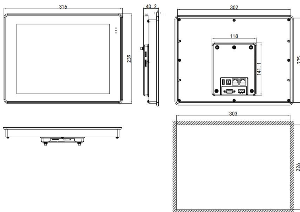
PI8121ig(N) 安装尺寸图
