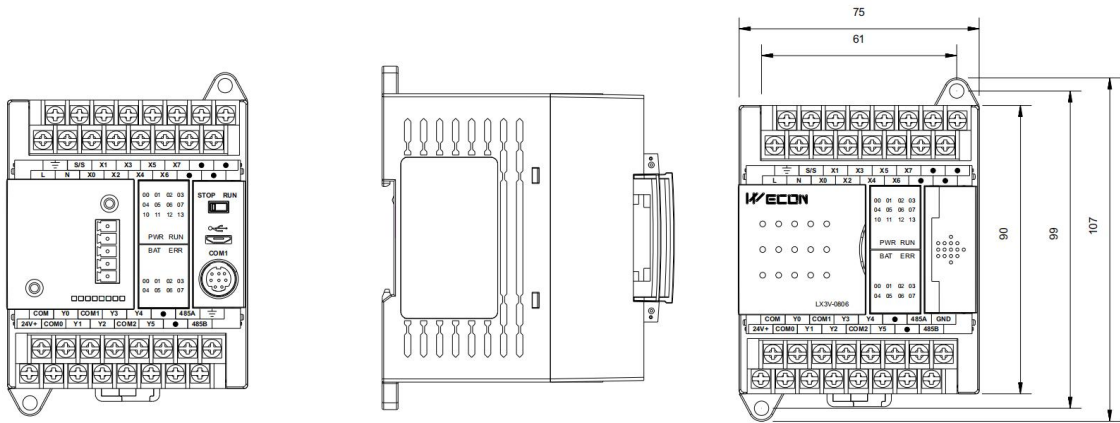
LX3V 0806 安装尺寸图
