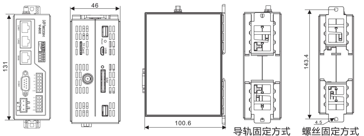
V-BOX H-00/H-WF/ H-4G/ H-AG 安装尺寸图
