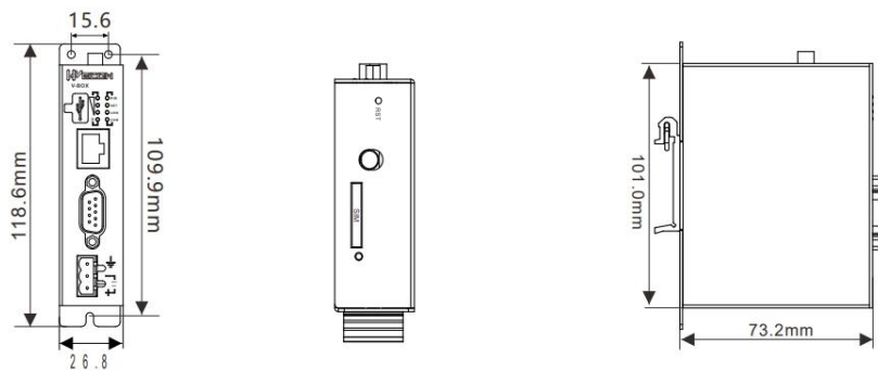
RE-00 / RE-4G 安装尺寸图
