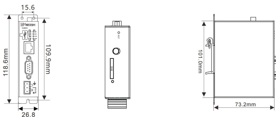
RE-00 / RE-4G 安装尺寸图
