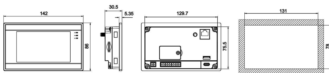
PI3043ig / PI8043ig 安装尺寸图
