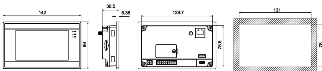
PI3043ig / PI8043ig 安装尺寸图
