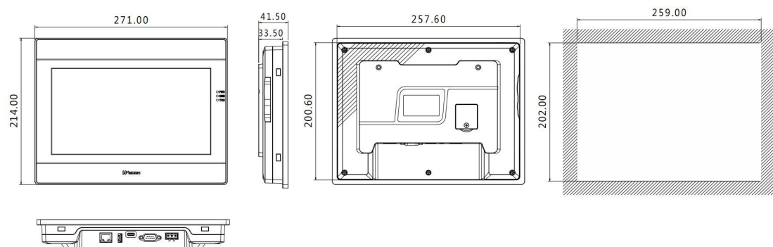
IN1101 安装尺寸图
