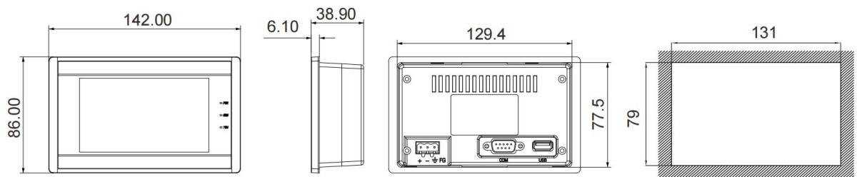
PI3043ie-T 安装尺寸图
