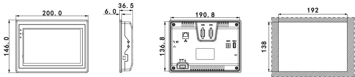
PI3070i-2S 安装尺寸图
