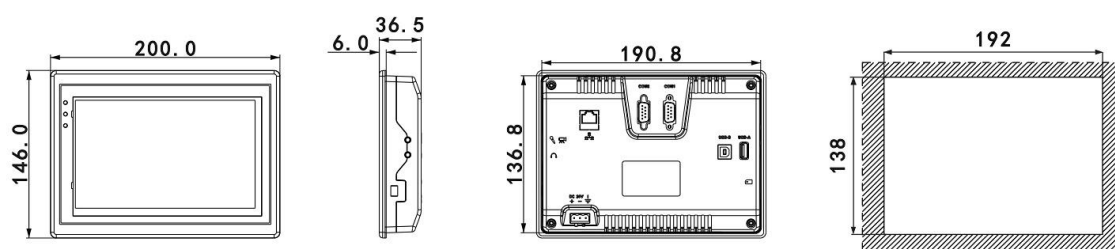
PI3070i-A 安装尺寸图
