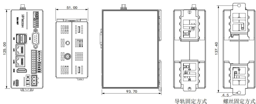
RH-WF 安装尺寸图
