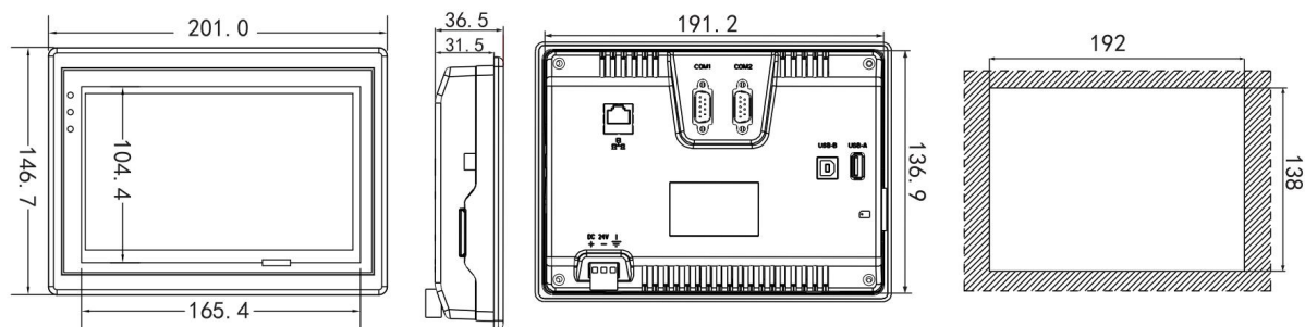
PI 8070/PI 8070C/PI 8070H 安装尺寸图
